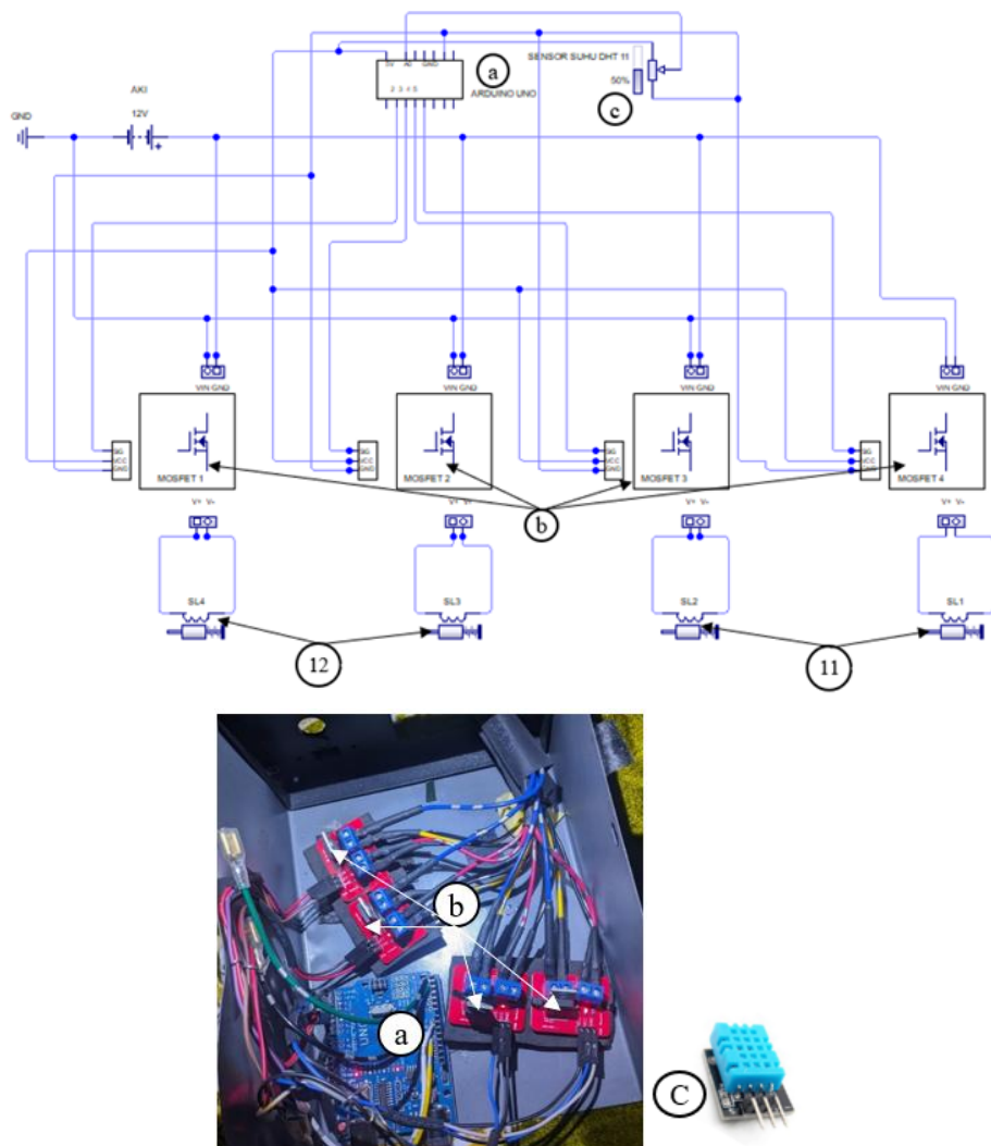
Fig. 2. ECU wiring diagram.
